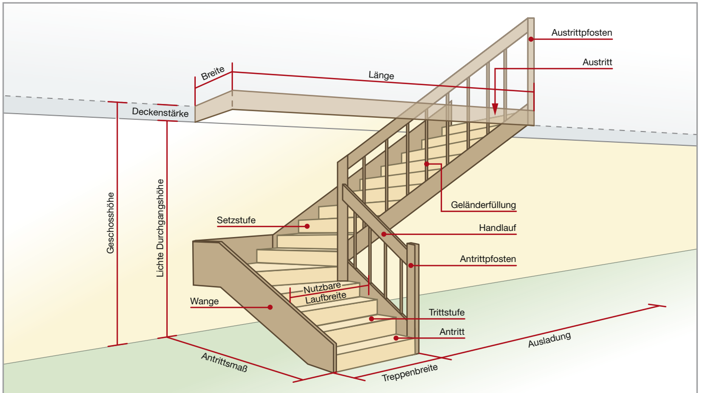
Elemente einer Treppe
